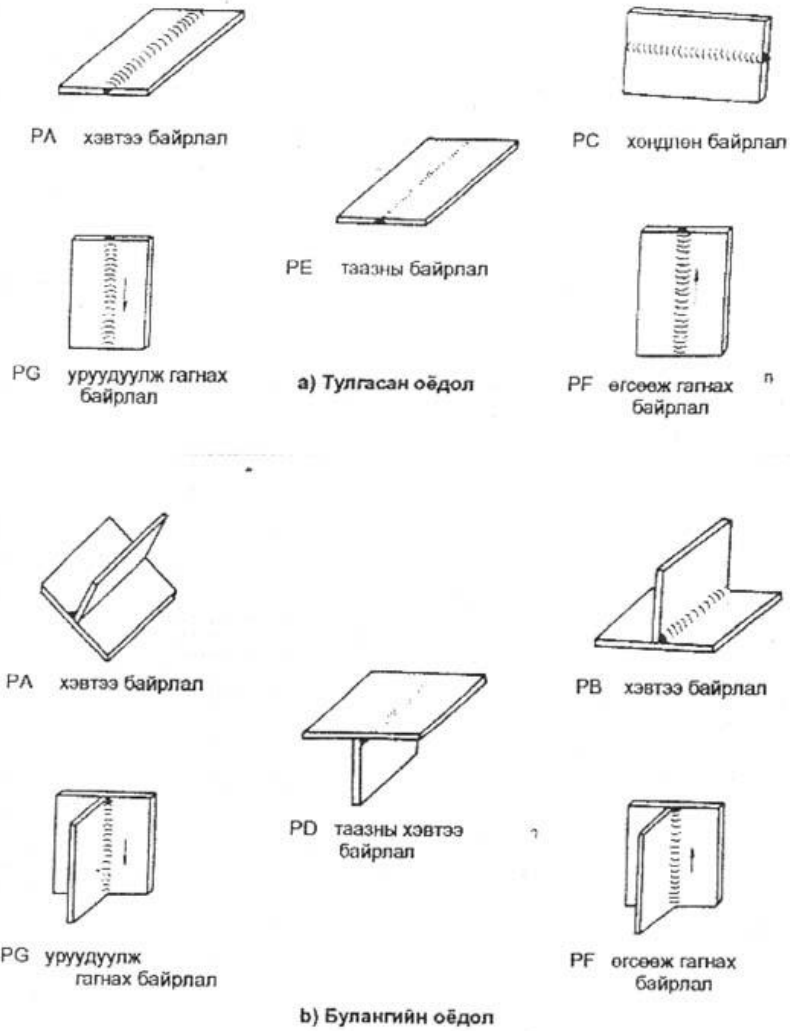
1-р зураг. Хавтан гагнах орон зайн байрлал
